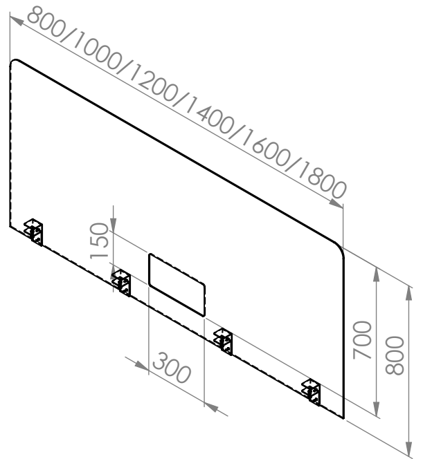
Divisória frontal com abertura
