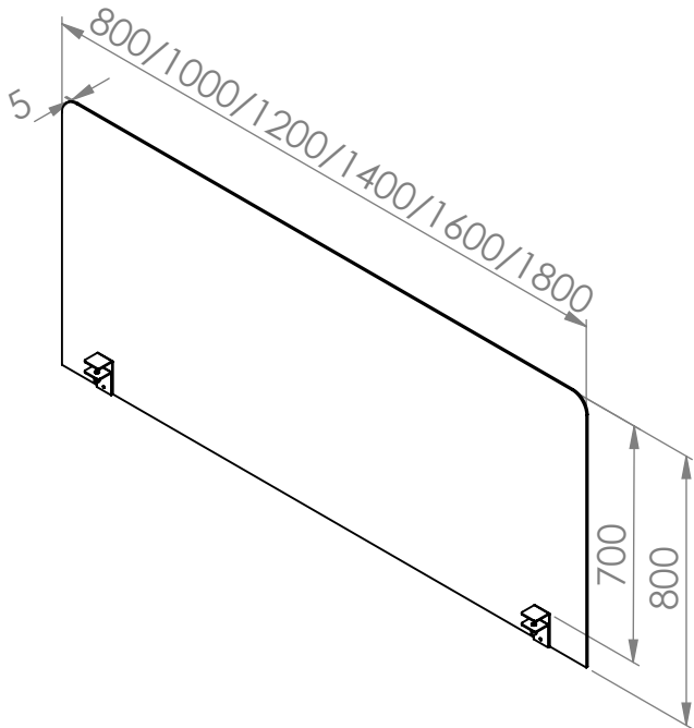
Divisória frontal sem abertura
