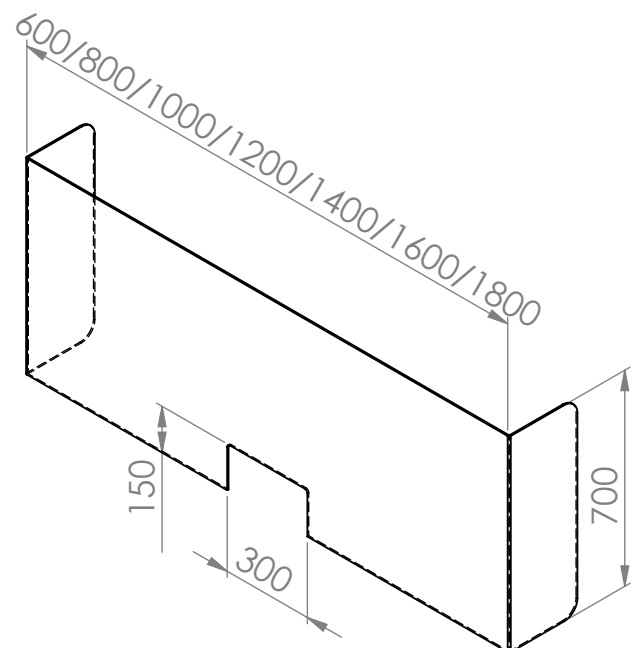
Divisória acrílica com abas com abertura
