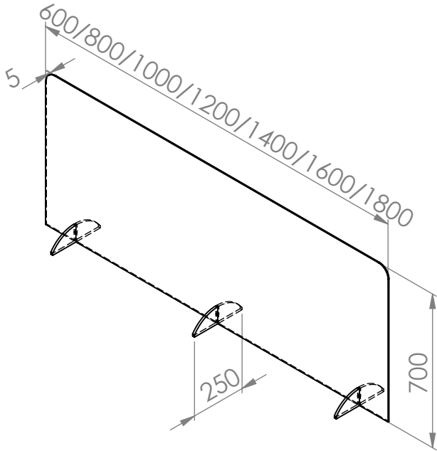
Divisória acrílica de pousar sem abertura
