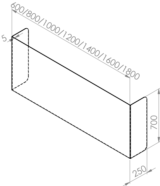
Divisória acrílica com abas sem abertura
