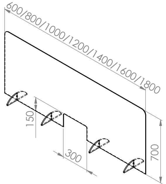
Divisória acrílica de pousar com abertura
