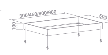
socos/zócalos
